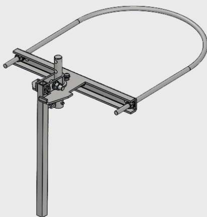
NNO - wersja dla żerdzi wirowanej
